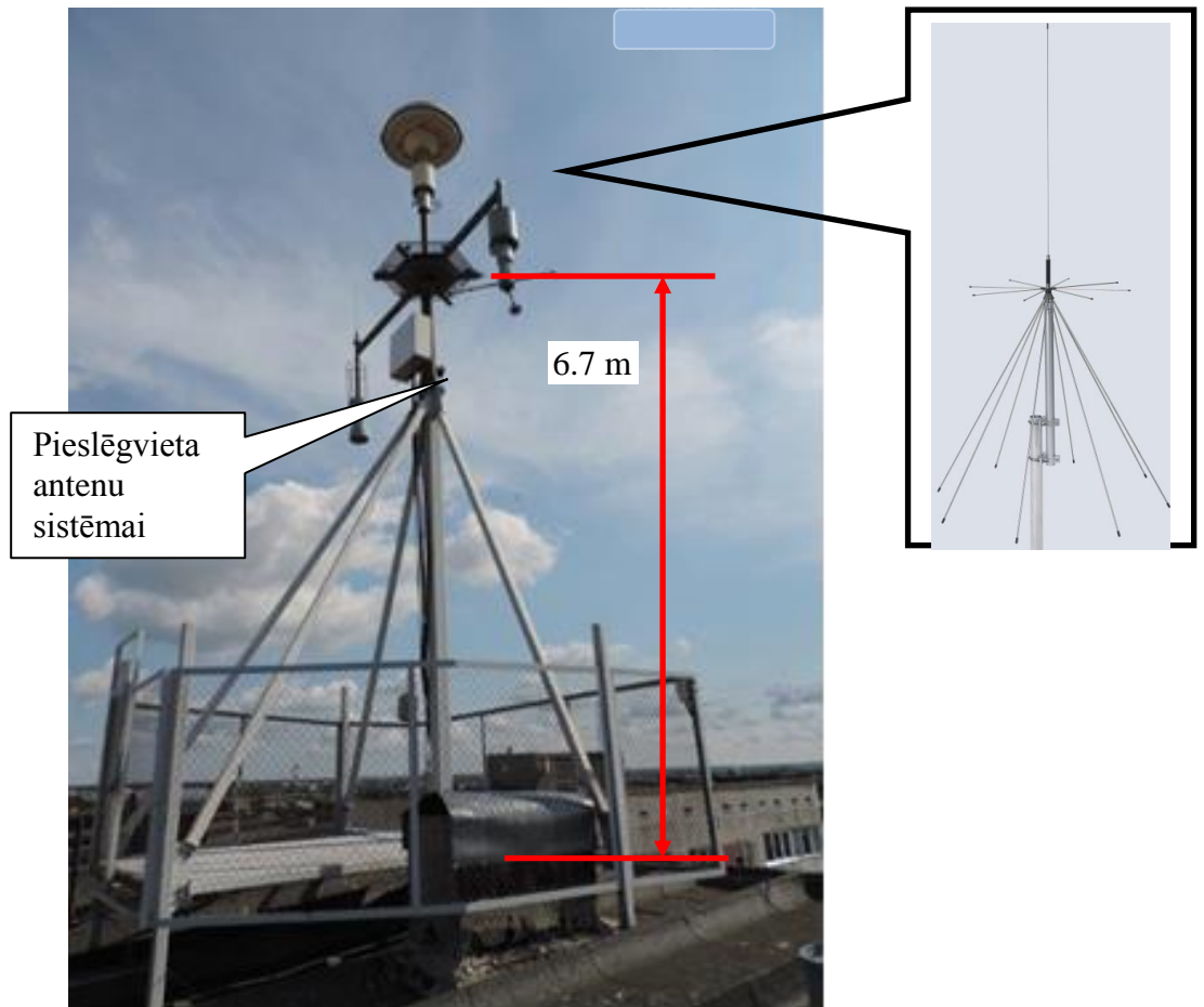
att.3 Platjoslas antenas uzstādīšana
