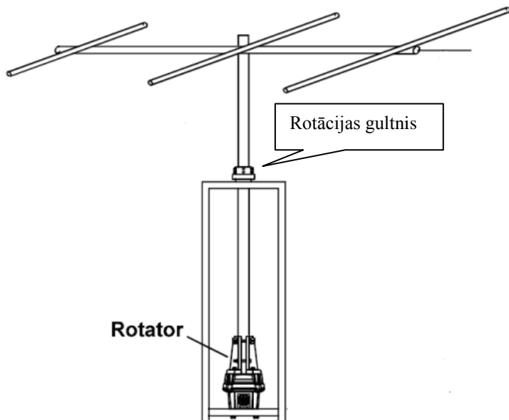
att.1 Pagriešanas mehānisma novietošana
